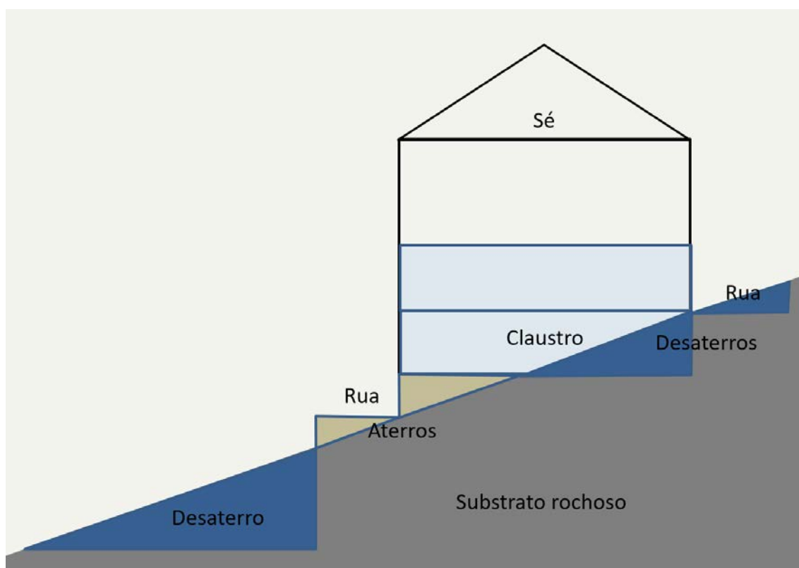
Figura 2 – Representação esquemática da manipulação do terreno no local de Sé de Lisboa, com a criação de plataformas artificiais através de desaterro – aterro construído.
